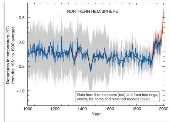
IPCC
